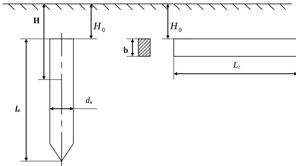
Рис. 1. Схема расположения электродов защитного заземления в грунте.
